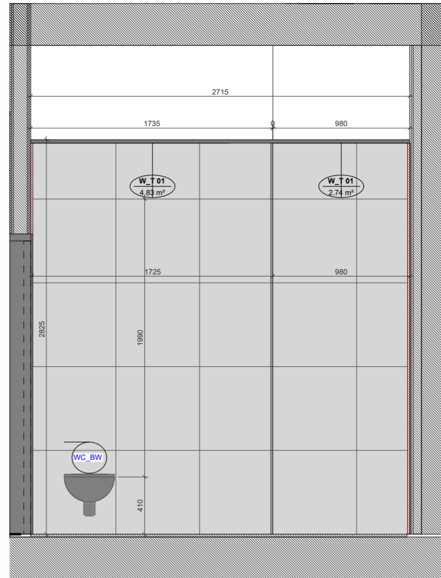
ELEVATION 1 1 : 25
